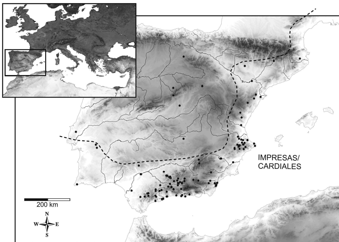
Figura 1. Mapa general del área de estudio con la distribución de sitios con brazaletes de piedra y en línea discontinua, culturas del Neolítico Antiguo caracterizadas por cerámicas decoradas cardiales e impresas
